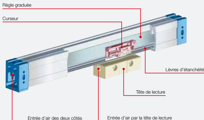
Codeur linéaire
