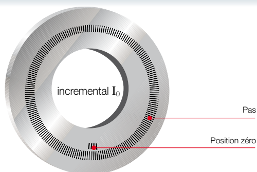
Codeur rotatif
