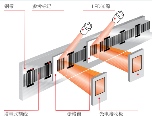
钢带光栅尺
