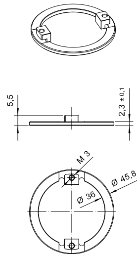
Arandela de exclusión de fallo mecánico W-35 W-35 mechanical fault exclusion washer Cod.: 82620158
