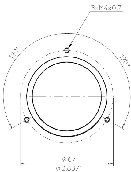
VISTA DEL SOPORTE BRACKET VIEW
